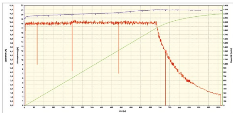
Ladeverlauf eines 5s-LiPo-Akkus mit 5.000 mAh Kapazität mit 10 A (2C)
