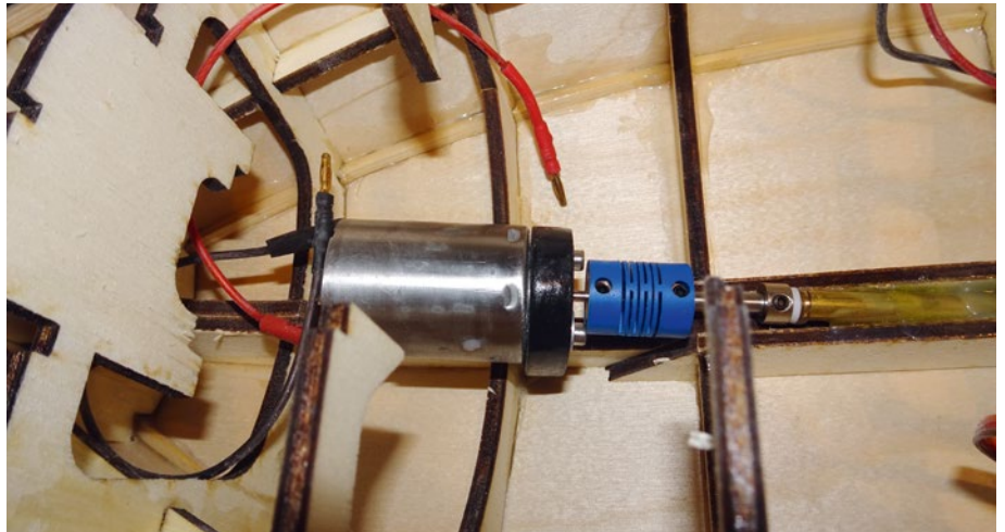
Die finale Verbindung zwischen Motor und Welle
