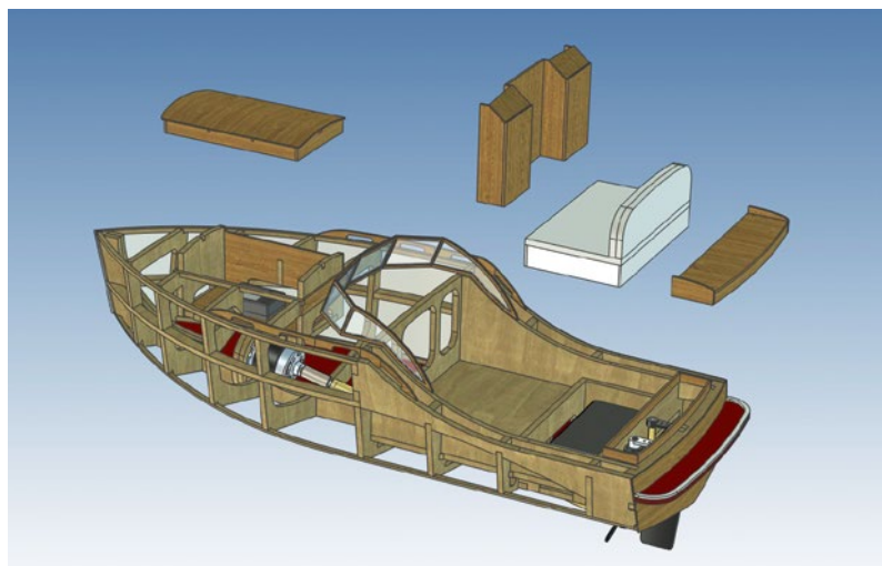
So wurde trotz der eigentümlichen Bauform des Backdeckers Zugang zu den Komponenten im Inneren geschaffen
