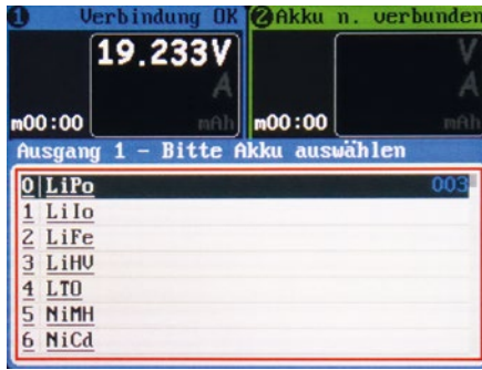
Zur Auswahl stehen eine Reihe Akkutypen, auch exotische wie LTO, also Lithium-Titanat-Oxid-Zellen mit 2,4 V pro Zelle
