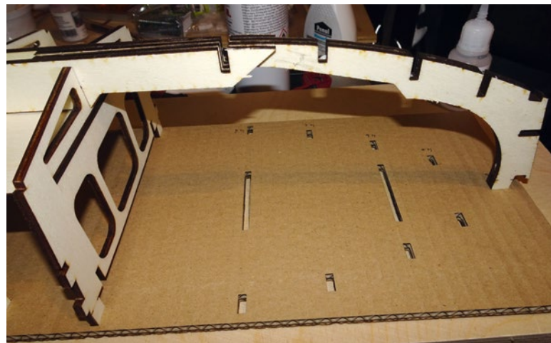
Der Kiel im Bugbereich. Die Helling besteht aus lasergeschnittener Pappe und sorgt für einen verzugsfreien Aufbau
