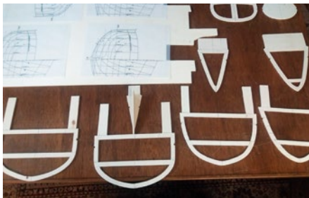
Die Spanten entstanden aus 5-mm-Pappelspertholz und sind zur Stabilisierung mit zusätzlichen Querstreben versehen
