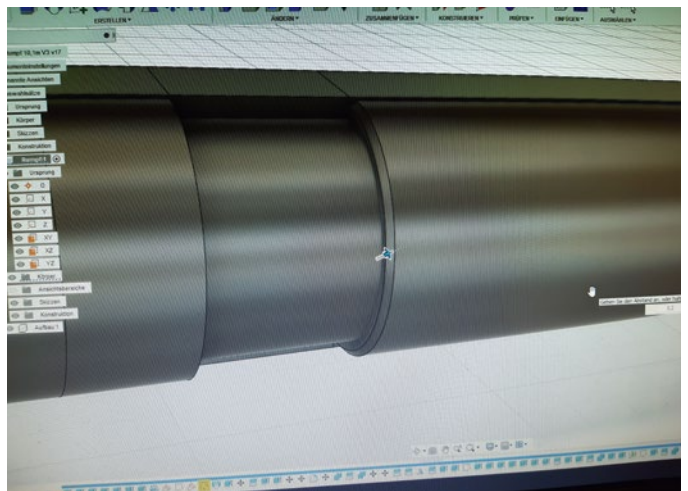
In einem zusätzlichen Schritt wurde der umlaufende Fender samt Aussparungen konstruiert
