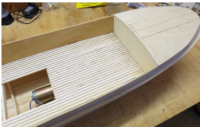
Das fertige Holzdeck und die Heckabdeckung. Gut ist hier die Innenverkleidung der Bordwände zu sehen
