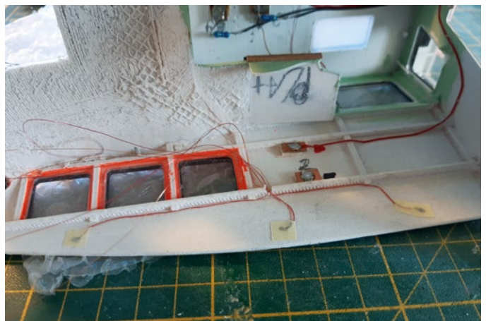
Für die Beleuchtung sind SMD mit Kupferlackdraht verbaut
