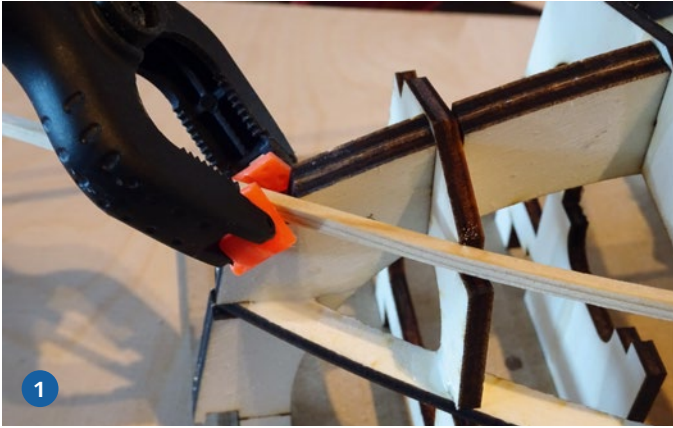
1) Die Stringer am Rumpfboden haben reichlich Spannung und müssen daher von einer resoluten Klammer gehalten werden, während der Kleber trocknet. 2) Das Spantengerüst im Heckbereich. Gut zu erkennen sind der Boden der Plicht und auch der Boden des Akkuraums. Vorsichtshalber wird jetzt schon das Verlängerungskabel zum Lenkservo eingezogen. Das Lenkservo ist ebenfalls schon installiert
