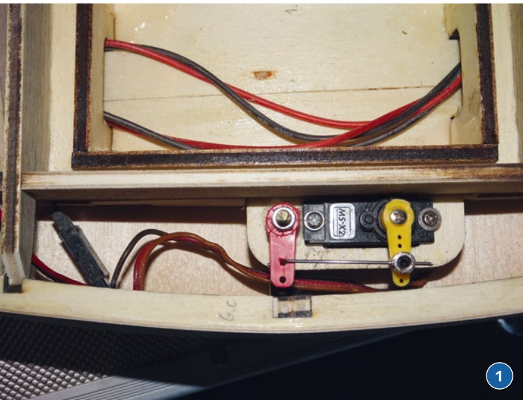
1) Kürzer und knackiger kann eine Ruderanlenkung nicht sein. 2) Diese beiden Konsolen bilden später zusammen mit einem Mittelteil die vordere Wand der Plicht. Auf dem Backdeck sind die gelaserten Linien für die Frontscheiben zu erkennen
