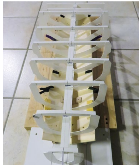
Das Spantengerüst wurde aus 1-mm-ABS-Platten erstellt
