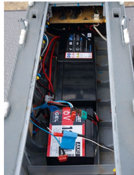
Platz für die drei Bleigel-Akkus ist bei der FRANKFURT AM MAIN ausreichend vorhanden. Und auch das Gewicht stellt kein Problem dar
