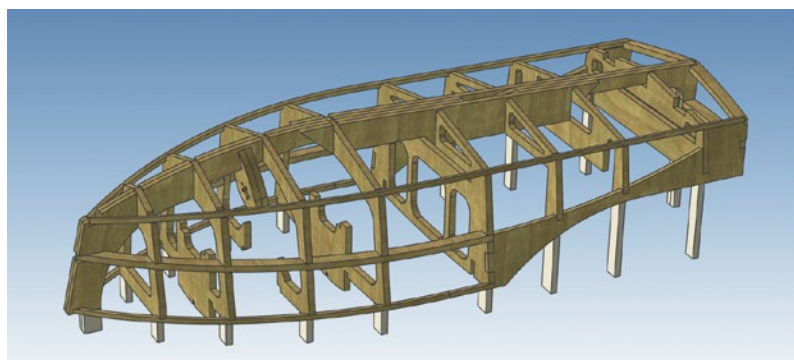
Das Spantengerüst wird über Kopf auf der Helling aufgebaut
