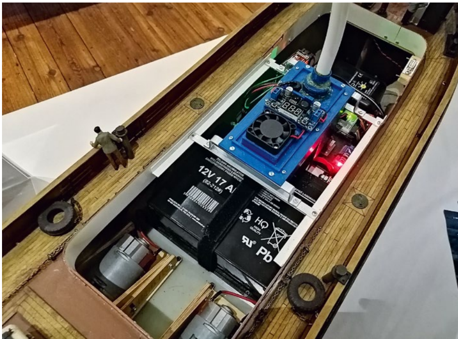
Blick in das Innenleben der IMARA. In der Mitte befindet sich der Rauchgenerator, vorne links unten die beiden einzeln ansteuerbaren Motoren
