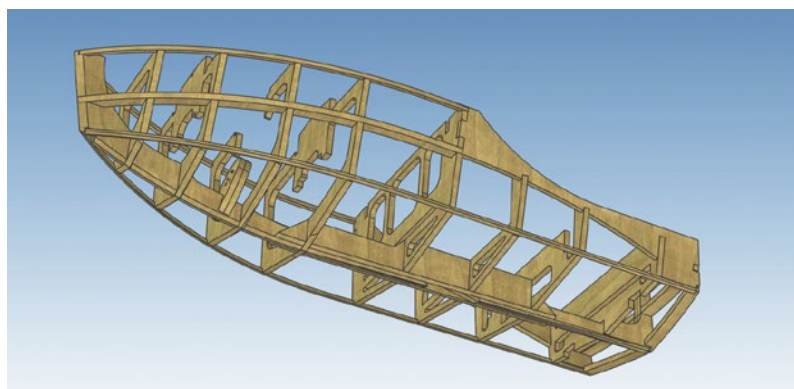
Der Knickspantrumpf wird aus dem Kiel, den Spanten und den Stringern zusammengesetzt
