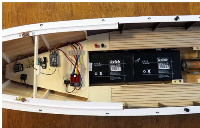
Bleiakkus verleihen der Barkasse Stabilität sowie das nötige Gewicht und sorgen für lange Fahrzeiten
