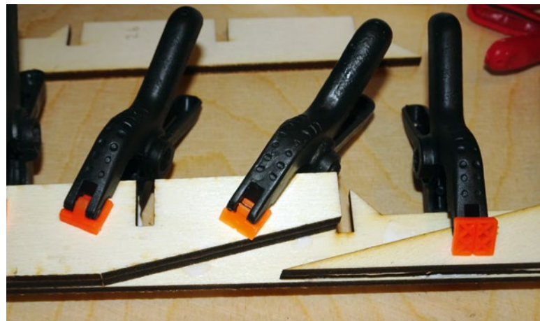
Der Kiel besteht aus mehreren Teilen, die zu Baubeginn miteinander verklebt werden. Gut zu erkennen, die Durchführung für das Stevenrohr ist schon konstruktiv vorbereitet
