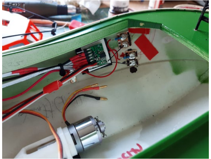
Nach dem Lackieren konnte mit dem technischen Ausbau begonnen werden
