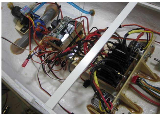
Unter Deck sind letztlich doch eine Reihe Antriebs, Zubehör-, RC- und Elektronikkomponenten unterzubringen
