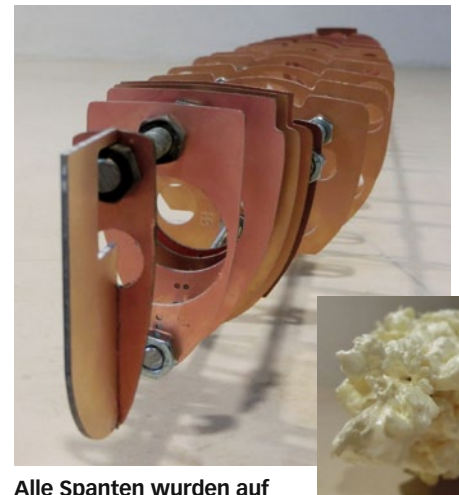
Alle Spanten wurden auf Gewindestangen aufgereiht und die Zwischenräume dann mit Bauschaum ausgefüllt. Letzterer war jedoch relativ weich, was sich beim anschließenden Spachteln als problematisch erwies
