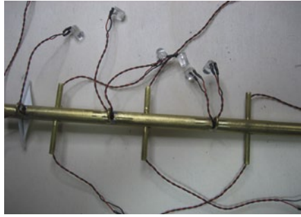
Eine Reihe Leitungen waren aufgrund der umfangreichen Beleuchtung im Mast unterzubringen
