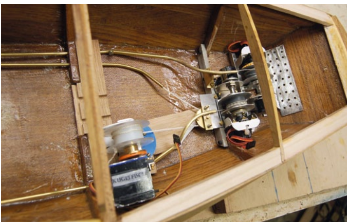
Die Schwert- und Großschotwinden an ihrem Einbauport. Die Führung der Seile erfolgt klassisch in Messingrohren
