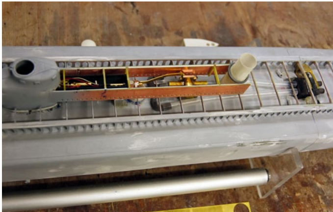
Blick auf Antrieb, Walze, Schornstein und Luftkupplung
