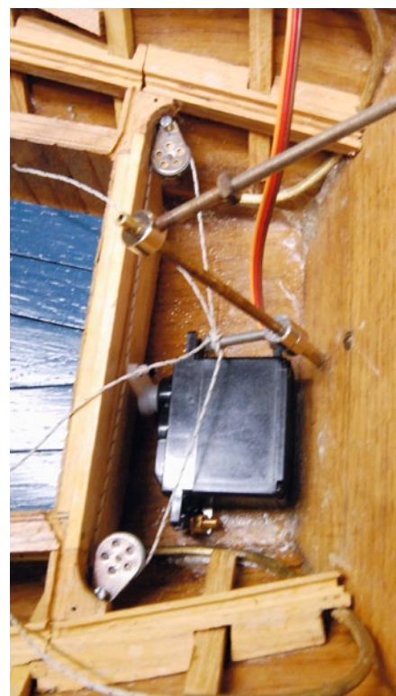
Über ein umlaufendes Seil lässt sich das schräge Ruder problemlos in beide Richtungen ziehen beziehungsweise bewegen
