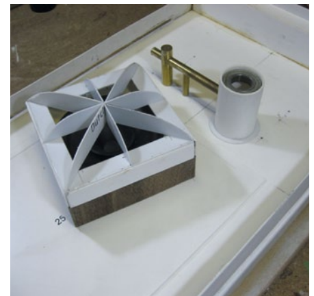
Blick auf die Kranaufgabe mit integriertem doppelten Kugellager und Durchführung der Energiezuführung der Kranbewegung
