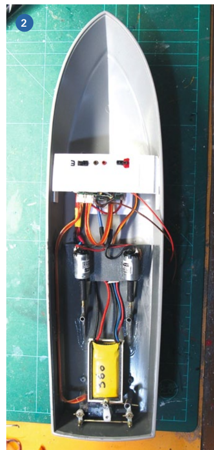
1) Die Wellenanlagen entstanden im Eigenbau, wobei die Wellen aus Silberdraht und die Rohre aus Messing sind. 2) Zwei noch vorhandene China-Noname-Motoren erhielten den Vorzug als Antriebsaggregate. 3) Ein sehr leichter Empfänger mit kleinen, leichten Steckkontakten ist Pflicht – ebenso der Thor-Regler. 4) Glücklicherweise fanden sich in einer Restekiste passende Propeller
