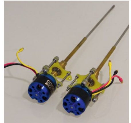
Motoren mit Halterungen, Kupplung, Stevenrohren und Antriebswellen
