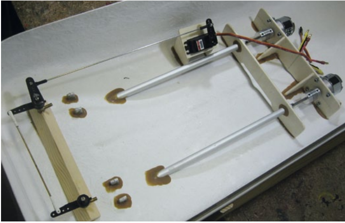
Einbau der Wellenanlage und Ruderansteuerung
