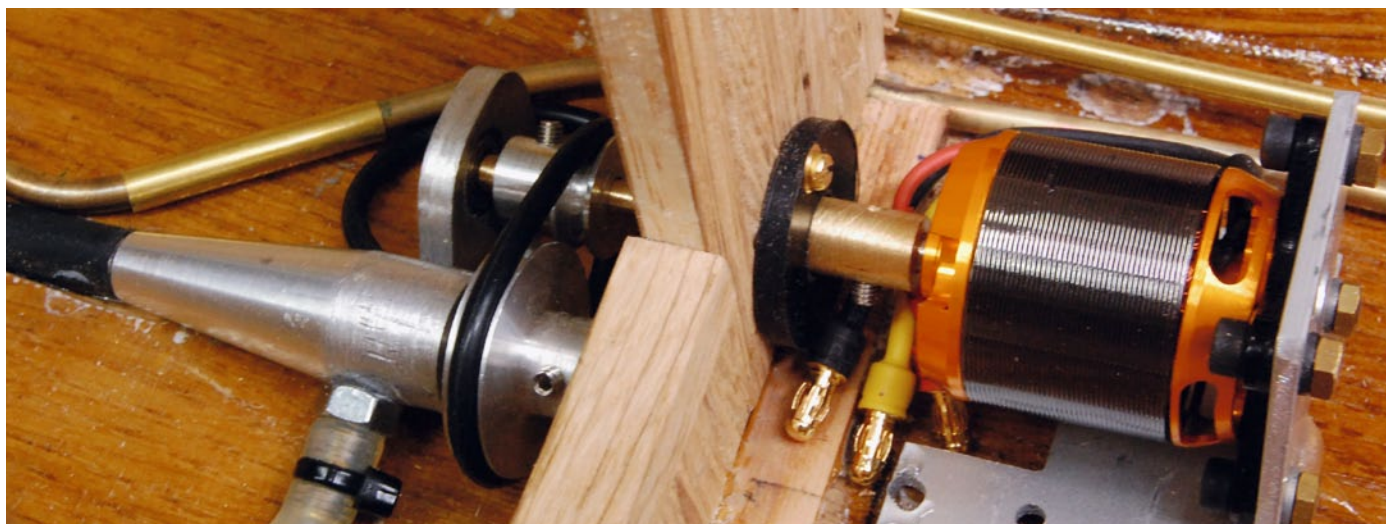
Der Betrieb über einen Riemen untersetzt einerseits die hohe Drehzahl und sorgt andererseits für eine gewisse Dämpfung sowie Sicherheit vor Blockaden
