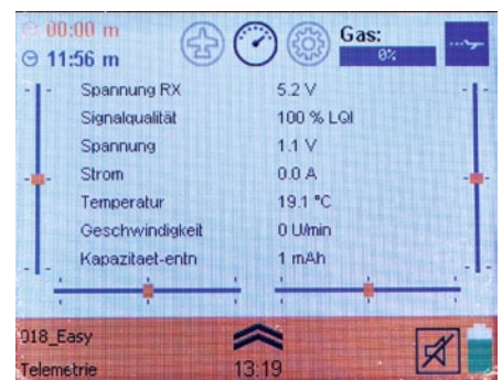
Telemetrieanzeige im Startmenü
