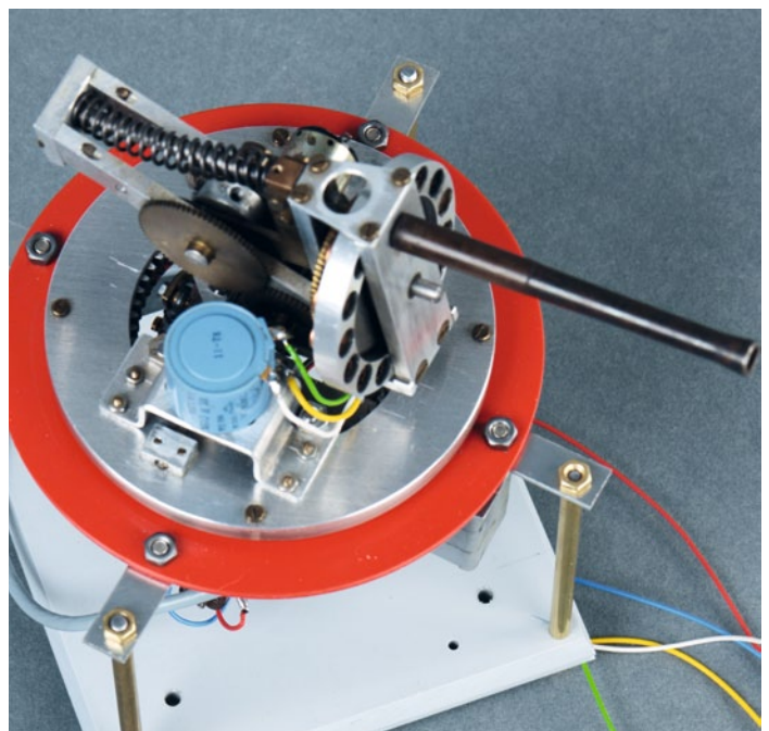
Die komplette Funktionseinheit mit montierter Kanone – ein Video dazu findet sich auf dem Youtube-Kanal von SchiffsModell
