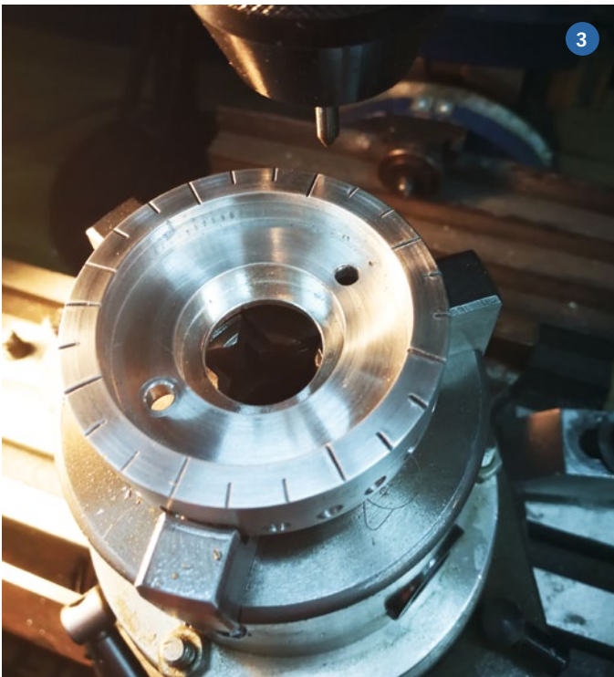
1) Grundkörper mit Nutensteinen. 2) Ausdrehen des Grundkörpers. 3) Gravieren der 24er-Teilung. 4) Vertikale Montage des selbst gestalteten Teilkopfs an der Proxxon MF 70
