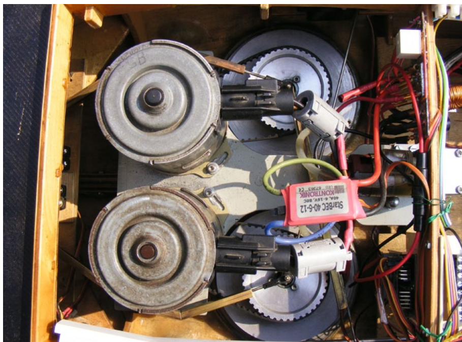
Blick auf die eingebauten VSP mit Motoren und Drehzahlsteller im Modell
