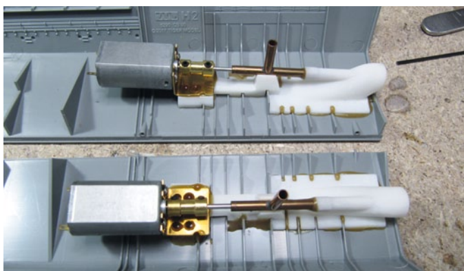
Die Jet-Antriebe aus China haben ihren Platz gefunden
