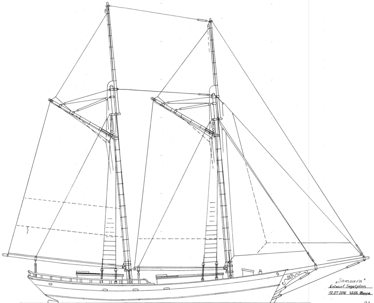
Blick auf den Segelriss der SAMSARA
