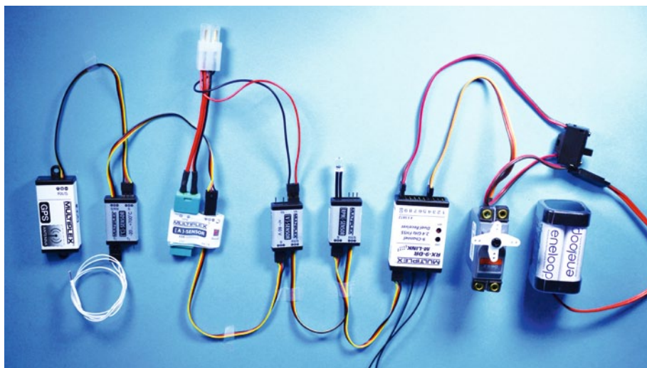
Die Empfänger mit Telemetriesensoren. Sie sind mit dem MPX-Launcher dann recht einfach den jeweiligen Adressen im Sender zuzuordnen
