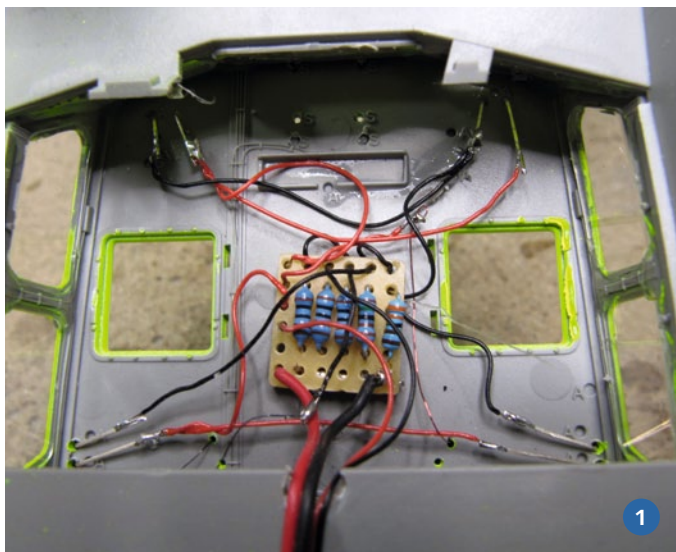
1) Für die Beleuchtung durch LED – Positionsbeleuchtung und Suchscheinwerfer – wurde diese Platine erstellt. Die blauen Widerstände sind mit farbigen Zahlen-Codes versehen, die den Widerstand angeben. Diese Vorwiderstände werden bei LED-Beleuchtungen benötigt. 2) Im Dunkeln wirkt die Beleuchtung natürlich besonders gut. 3) Da beide Motoren nicht wirklich synchron beschleunigen, ist regelmäßiges Nachregeln nötig. 4) Der 2,4-Gigahertz-Empfänger befindet sich gut zugänglich unter der nicht benötigten Maschinengewehr-Abdeckung vor dem Steuerhaus
