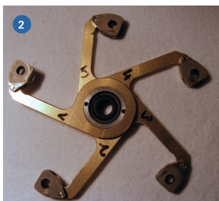
1) Alle Elemente des zu Wartungszwecken demontierten Voith Schneider Propeller-Antriebs mit den neuen Lenkern. 2) Steuer-scheibe mit aufgesteckten neuen Lenkern und Messerhebeln, ohne Deckelscheibe. 3) Steuerscheibe aufgepresst auf Schwenklager und Deckelscheibe
