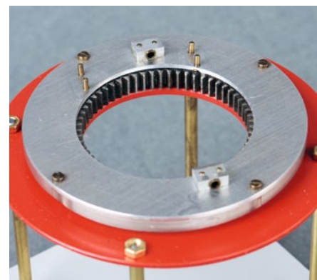
Der Auflagering zentriert sich auf dem Zahnkranz
