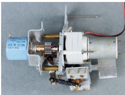
Die Antriebseinheit: Getriebemotor, Zahnrad und Poti auf einer Wellenkupplung
