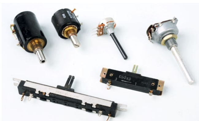
Potis dienen uns als Lagegeber, es gibt sie in unterschiedlichen Bauformen
