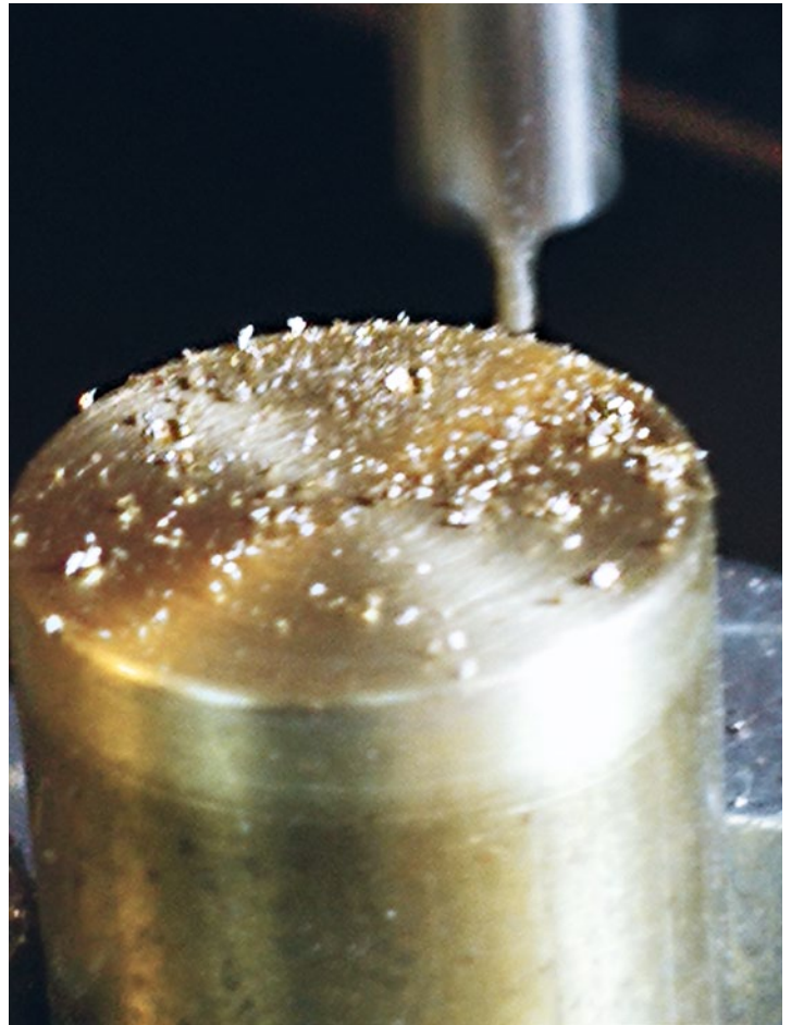
Zwei Versuche mit dem neuen Mini-Teilkopf. Nun kann ganz nach den eigenen Bedürfnissen gefräst werden
