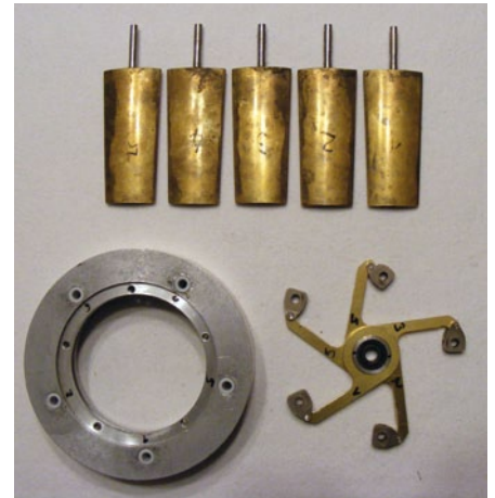
Fertiger Messersatz aus Teppichschienen. Rotor mit Teflongleitlagern (unten links). Steuerscheibe mit neuen Lenkern und montierten Messerhebeln
