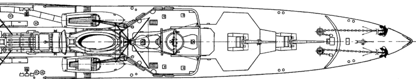
Generalplan M 1:350
