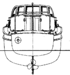
er-Pinasse (sd126) M 1:100
