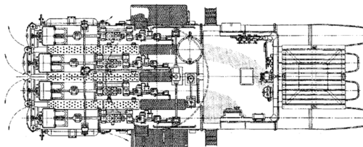
533-mm-TR-Vierling (sd026) M 1:100
