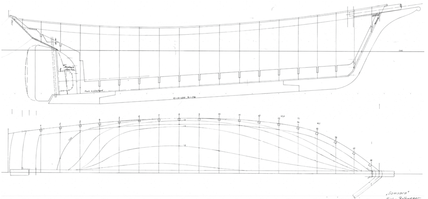
Seiten- und Draufsicht inklusive Kielform
