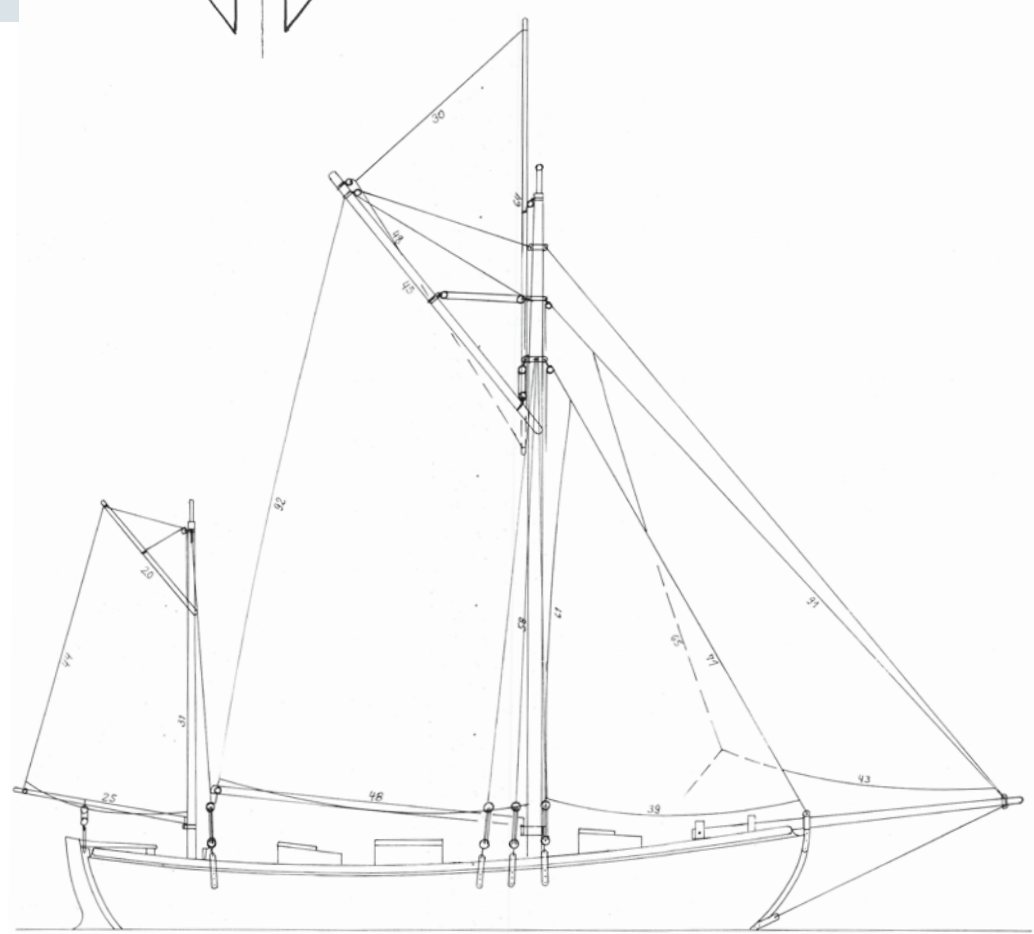
COLIN ARCHER RS1 Segelplan M. 1:36 14.12.2013 Willi Röpcke
