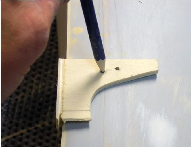
Kleine Helferlein erleichtern das Anzeichnen ungemain
