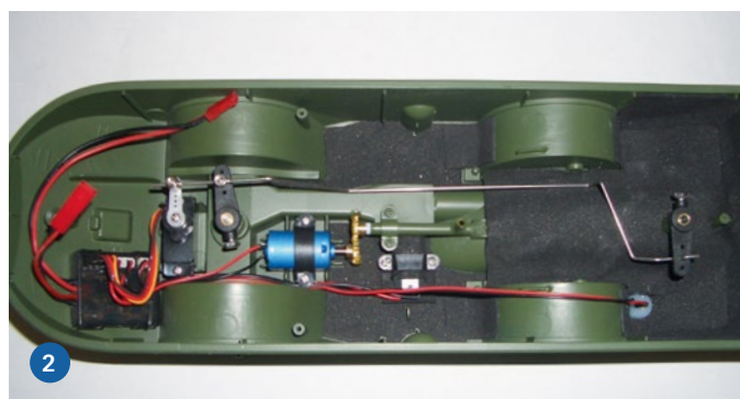
1) Der extra angeschaffte Fahrer muss erstmal zusammengesetzt werden. 2) Auch der Fahrerraum lässt sich abschrauben und gibt einen Blick in die Unterwanne frei: Mit einem Gestänge wird das Steuerruder im Heck angelenkt. Die schwarzen Moosgummimatten dienen als Schallschutz
