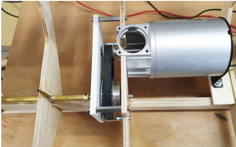
Um die Drehzahl zu reduzieren und das Drehmoment zu erhöhen, ist der Heckantrieb mit einem Riemengetriebe untersetzt
