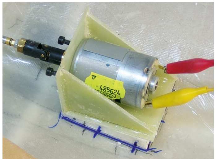
Der entnehmbare Motorhalter erlaubt Wartungsarbeit in zwei Minuten
