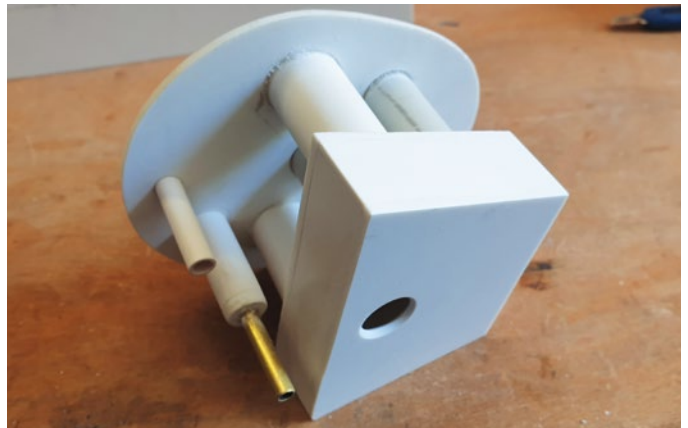
Im Schornstein ist ein Rauchgenerator installiert. Über die Box verteilt sich der Rauch auf vier Schlotte
