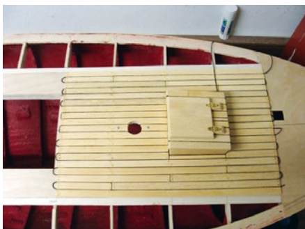
Eine Möglichkeit zum Andeuten der Kalfaterung sind eingelassene Fäden
