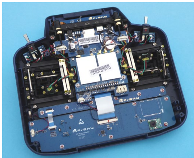
Professionelle Technik wird sichtbar, wenn der Sender geöffnet wird
