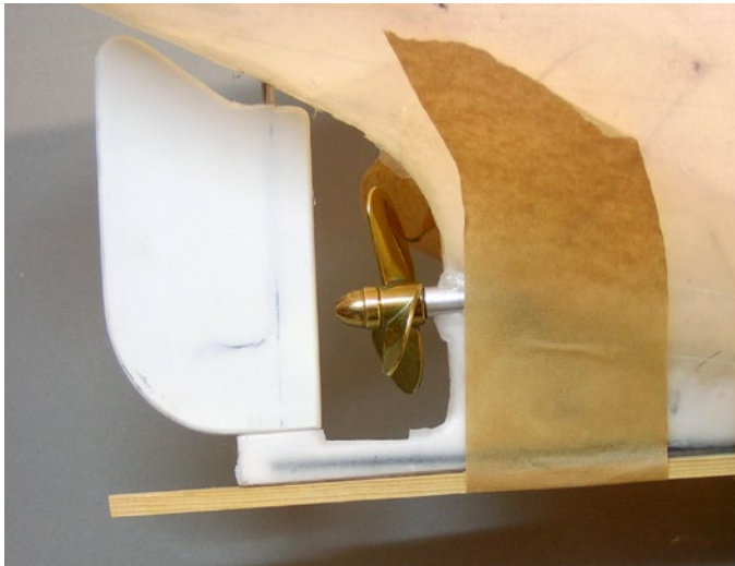
Ruder und Schiffspropeller. Wichtig: Der Schutz der Ruderhacke während des Baus
