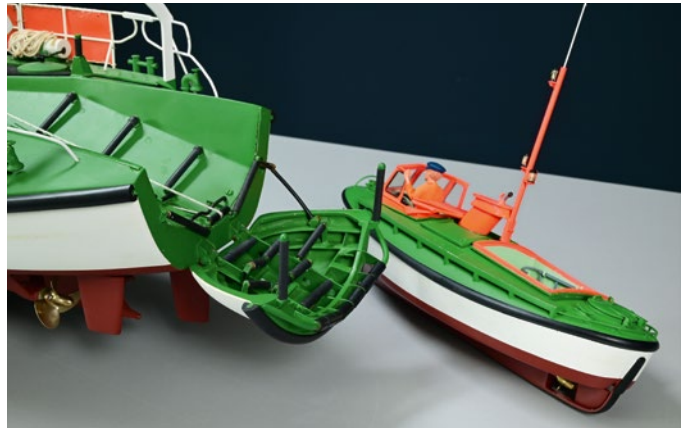
Die Heckklappe wurde 2002 neu gebaut, aber die Mechanik und Antriebe zur Ansteuerung sind seit den 1980er-Jahren im Betrieb
