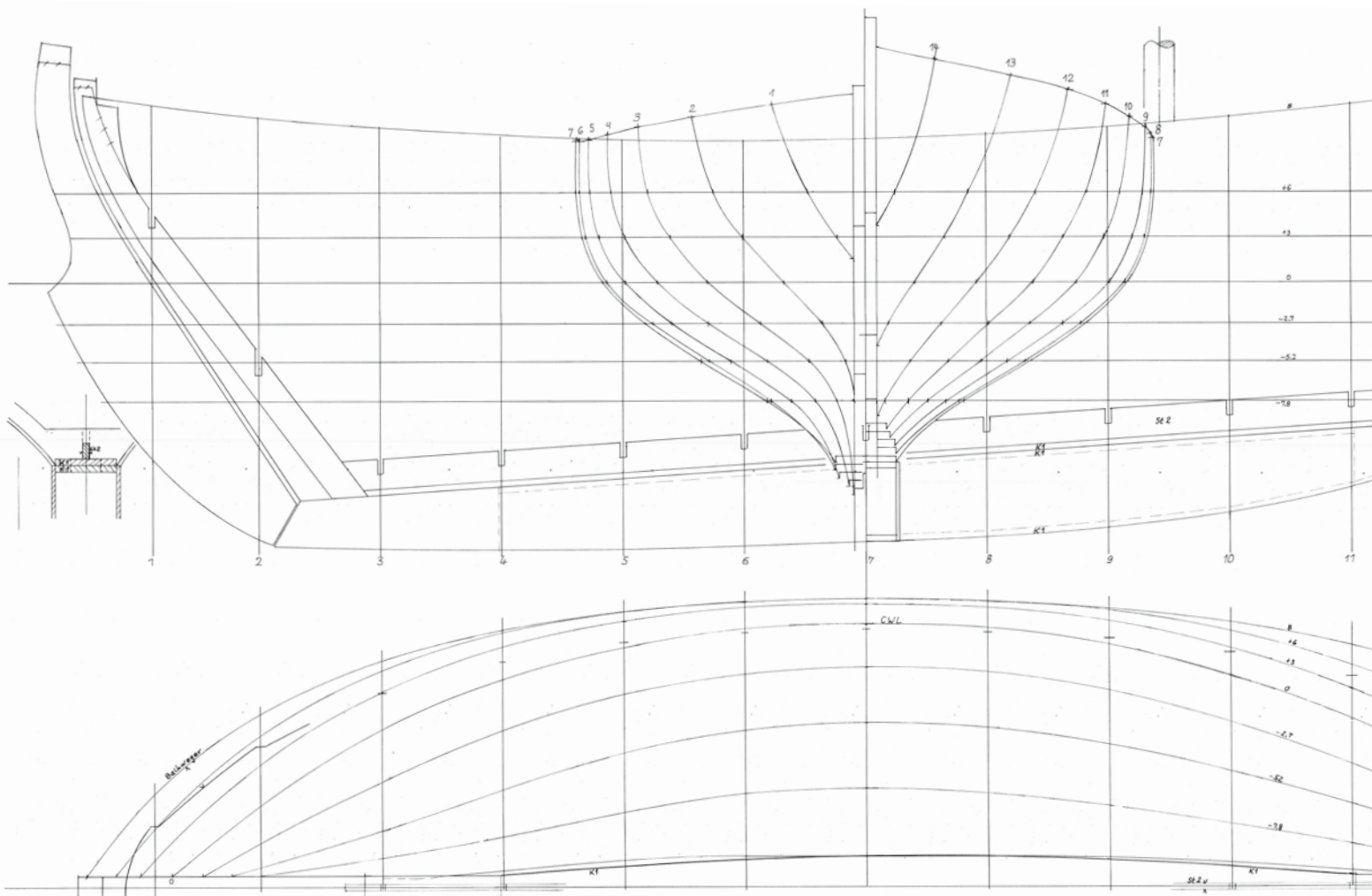
Spanten, Steven, Bug und Kiel sind anhand der Bauplanskizze zu fertigen
