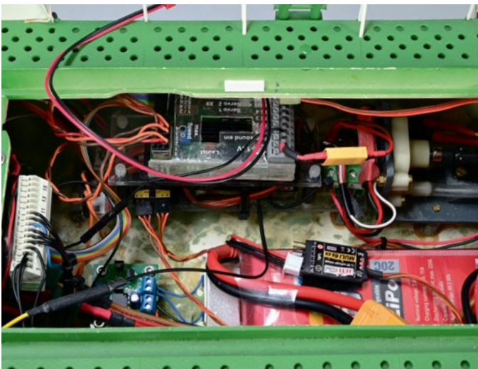
Neue Motoren, Regler, Akku und ein Beier-Modul zogen beim jüngsten Refit ins Rumpffinnere ein
