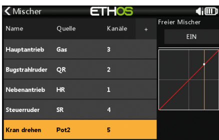
Im Überblick könnten sich die angelegten Mischer so darstellen
