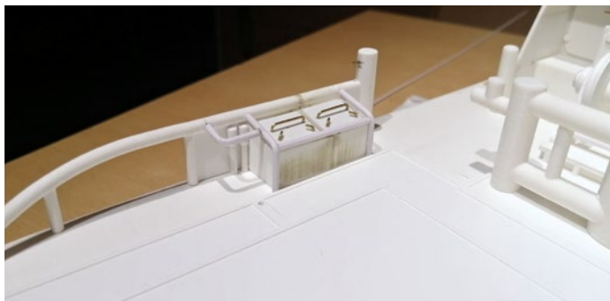
Mit Hilfe von Fotos eines möglichen Originals wurden zahlreiche Details an Deck ergänzt
