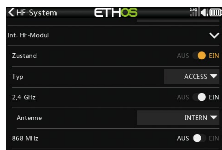
Die HF-Module für beide Funkstrecken lassen sich übersichtlich konfigurieren
