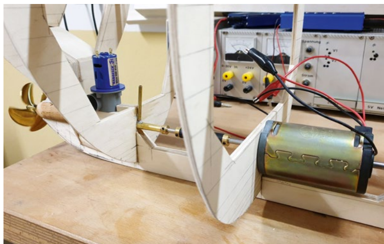
Der Motoreinbau, vorne und hinten, erfolgte zu einem frühen Zeitpunkt, um alles exakt justieren zu können – hier der Bugmotor mit Querstrahler
